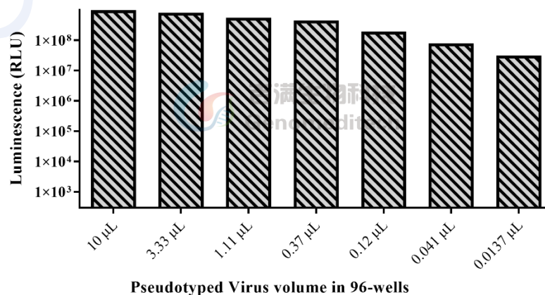
图2 吉满 SARS-CoV-2 Spike S 蛋白(LB.1)突变型假病毒感染 HEK293T-ACE2 测定 Luciferase 数值
